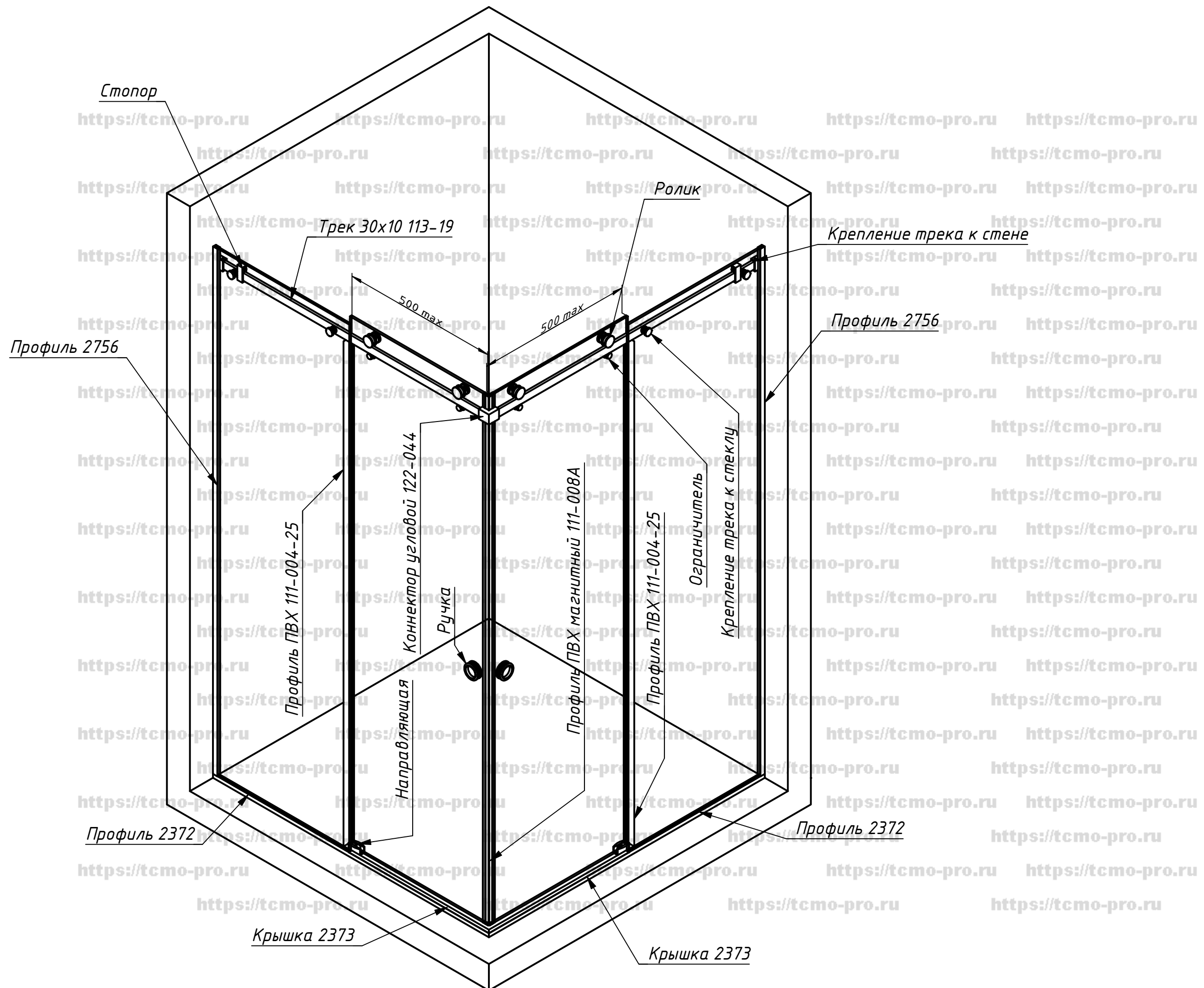
Схема угловой душевой кабины из 2-х комплектов 133-002
